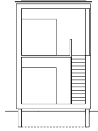
QUERSCHNITT | DIE ZWEIFESCHOSSIGE TREPPENZEONE VERLEIHT DEM KLEINHAUS EINE GEWISSE GROSSZÜGIGKEIT.
