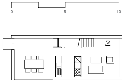
GRUNDRISS ERDGESCHOSS | DER KÜCHEN- BLOCK IM ZENTRUM ZONIERT DAS GE- SCHOSS IN ZWEI BEREICHE
