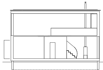
LÄNGSSCHNITT | JEDER RAUM RICHTET SICH MIT EINEM GROSSEN FENSTER IN JE EINE HIMMELSRICHTUNG
